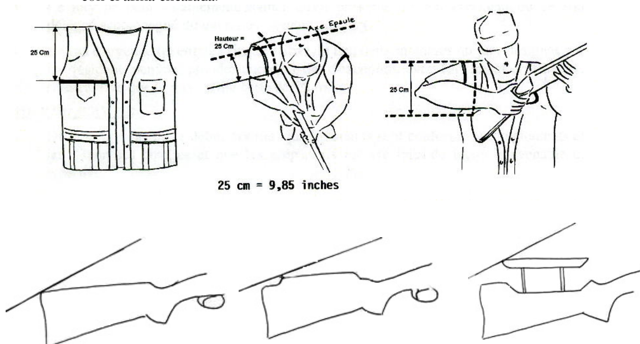
Culatas estándar
